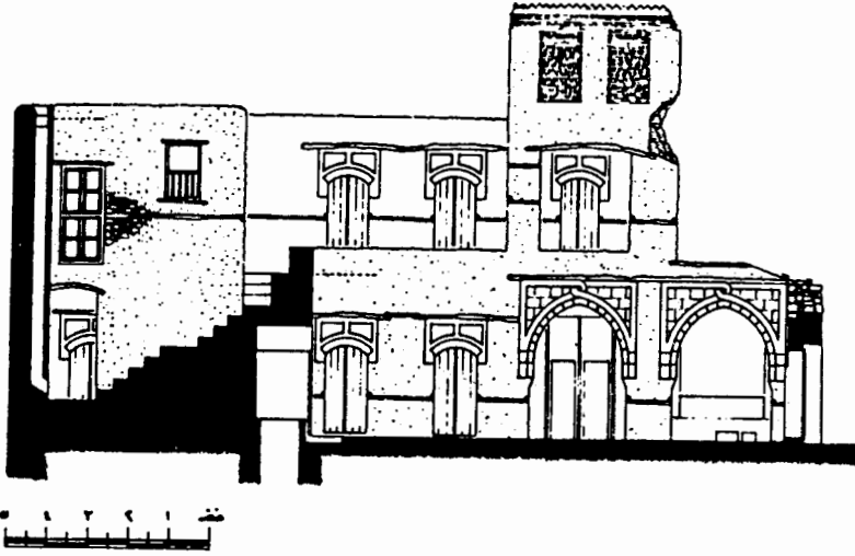
رباط الخيل : مقطع (نقلًا عن أولانكين)
